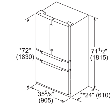
B36CL80ENS Dimensions
