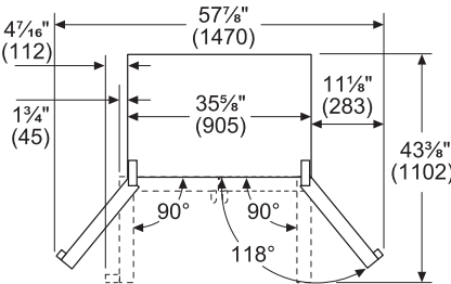
B36CT81SNS (Overhead Views)
