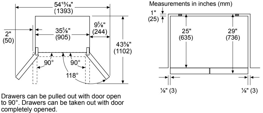
B36CL81ENG Dimensions (Overhead Views)
