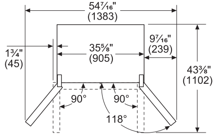
B36CL80ENS (Overhead Views)
